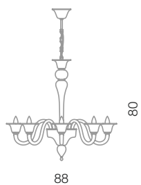
Barena lampadario 8L L 88 cm - H 80 cm 8 x E14 40W
