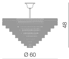
Mosca sospensione Ø 60 cm Ø 60 cm - H 48 cm 6 x E14 40W
