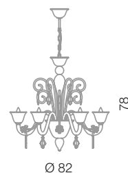
Alvis lampadario 6L Ø 82 cm - H 78 cm 6 x E14 40W
