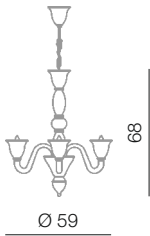
Laguna lampadario 4L Ø 59 cm - H 68 cm 4 x E14 40W
