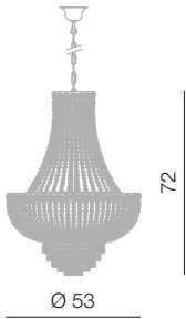
Amsterdam lampadario Impero Ø 50 cm Ø 53 cm - H 72 cm 7 x E14 40W
