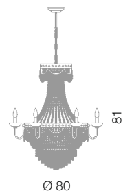
Pegaso lampadario Impero Ø 55 cm Ø 80 cm - H 81 cm 13 x E14 40W
