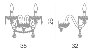
Toledo parete 2L L 35 cm - H 26 cm - SP 32 cm 2 x E14 40W
