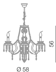
Alicante lampadario 4L Ø 58 cm - H 56 cm 4 x E14 40W
