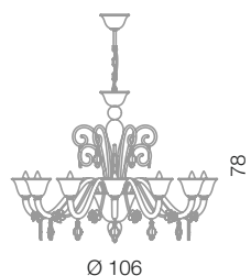
Alvis lampadario 12L Ø 106 cm - H 78 cm 12 x E14 40W
