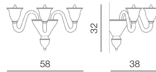
Laguna parete 3L L 58 cm - H 32 cm - SP 38 cm 3 x E14 40W
