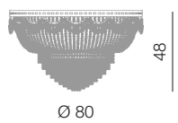
Pegaso plafoniera Ø 80 cm Ø 80 cm - H 48 cm 12 x E14 40W
