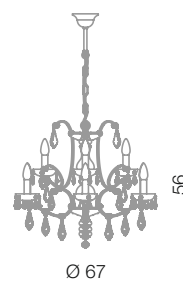
Salisburgo lampadario 6+3L Ø 67 cm - H 56 cm 9 x E14 40W
