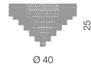
Mosca plafoniera Ø 40 cm Ø 40 cm - H 25 cm 3 x E14 40W
