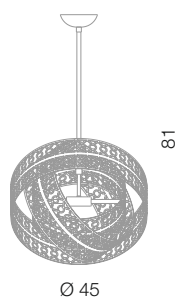
Galaxy lampadario 4L Ø 45 cm - H 81 cm 4 x G9 40W
