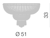
Beethoven plafoniera Ø 50 cm Ø 51 cm - H 33 cm 6 x E14 40W
