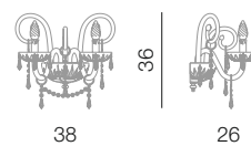
Erika parete 2L L 38 cm - H 36 cm - SP 26 cm 2 x E14 40W
