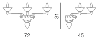
Ca' d'Oro parete 3L L 72 cm - H 31 cm - SP 45 cm 3 x E14 40W
