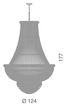
Osaka lampadario Impero Ø 120 cm Ø 124 cm - H 177 cm 20 x E14 40W
