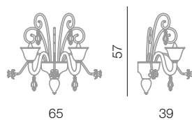
Alvis parete 2L L 65 cm - H 57 cm - SP 39 cm 2 x E14 40W
