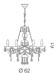
Serenade lampadario 6L Ø 62 cm - H 61 cm 6 x E14 40W
