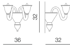
Laguna parete 2L L 36 cm - H 32 cm - SP 32 cm 2 x E14 40W
