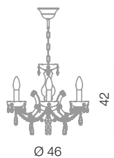
Vienna lampadario 3L Ø 46 cm - H 42 cm 3 x E14 40W
