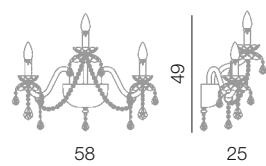
Temptation parete 3L L 58 cm - H 49 cm - SP 25 cm 3 x E14 40W
