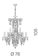
Dream lampadario 8+4L Ø 76 cm - H 105 cm 12 x E14 40W
