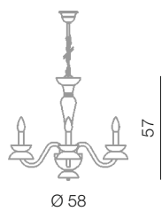
Dalí lampadario 4L Ø 58 cm - H 52 cm 4 x E14 40W
