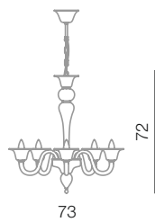
Barena lampadario 5L L 73 cm - H 72 cm 5 x E14 40W
