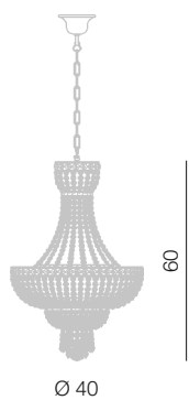
Beethoven lampadario Impero Ø 40 cm Ø 40 cm - H 60 cm 6 x E14 40W
