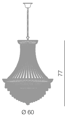
New Orleans lampadario Impero Ø 60 cm Ø 60 cm - H 77 cm 9 x E14 40W
