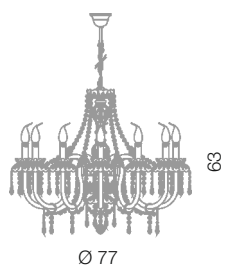
Alicante lampadario 12L Ø 77 cm - H 63 cm 12 x E14 40W
