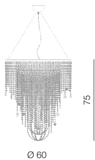
Cascade lampadario Ø 60 cm Ø 60 cm - H 75 cm 9 x E14 40W
