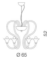
Babylon lampadario 6L Ø 65 cm - H 52 cm 6 x E14 40W
