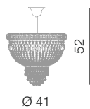
Osaka sospensione Ø 40 cm Ø 41 cm - H 52 cm 4 x E14 40W
