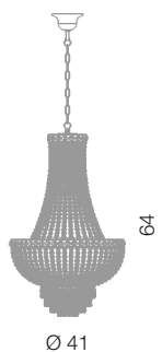
Settat lampadario Impero Ø 40 cm Ø 41 cm - H 64 cm 6 x E14 40W
