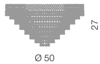
Mosca plafoniera Ø 50 cm Ø 50 cm - H 27 cm 4 x E14 40W
