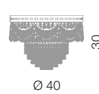
Pegaso plafoniera Ø 40 cm Ø 40 cm - H 30 cm 4 x E14 40W
