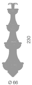
Osaka lampadario Impero MULTI Ø 66 cm Ø 66 cm - H 230 cm 21 x E14 40W
