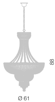
Beethoven lampadario Impero Ø 60 cm Ø 61 cm - H 88 cm 9 x E14 40W
