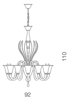
Rialto lampadario 12L L 92 cm - H 110 cm 12 x E14 40W
