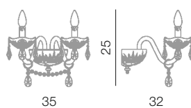
Siviglia parete 2L L 35 cm - H 25 cm - SP 32 cm 2 x E14 40W
