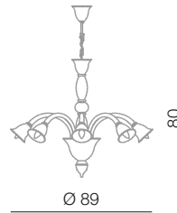
Laguna lampadario 8L BB Ø 89 cm - H 80 cm 8 x E14 40W
