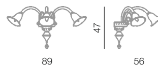
San Marco parete 3L L 89 cm - H 47 cm - SP 56 cm 3 x E14 40W
