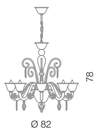
Alvis lampadario 8L Ø 82 cm - H 78 cm 8 x E14 40W
