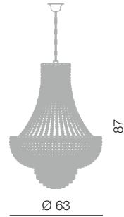
Amsterdam lampadario Impero Ø 60 cm Ø 63 cm - H 87 cm 9 x E14 40W
