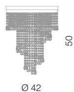
Twister plafoniera Ø 40 cm Ø 42 cm - H 50 cm 7 x E14 40W
