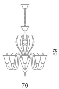
Rialto lampadario 8L L 79 cm - H 89 cm 8 x E14 40W
