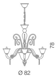
Alvis lampadario 4L Ø 82 cm - H 78 cm 4 x E14 40W
