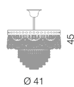
Pegaso sospensione Ø 40 cm Ø 41 cm - H 45 cm 4 x E14 40W
