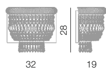
Osaka parete 3L L 32 cm - H 28 cm - SP 19 cm 3 x E14 40W
