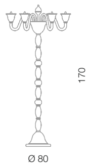
Laguna piantana 6L Ø 80 cm - H 170 cm 6 x E14 40W
