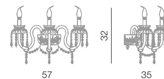
Alicante parete 3L L 57 cm - H 32 cm - SP 35 cm 3 x E14 40W
