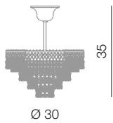
Mosca sospensione Ø 30 cm Ø 30 cm - H 35 cm 3 x E14 40W
