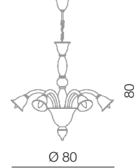
Laguna lampadario 6L BB Ø 80 cm - H 80 cm 6 x E14 40W
